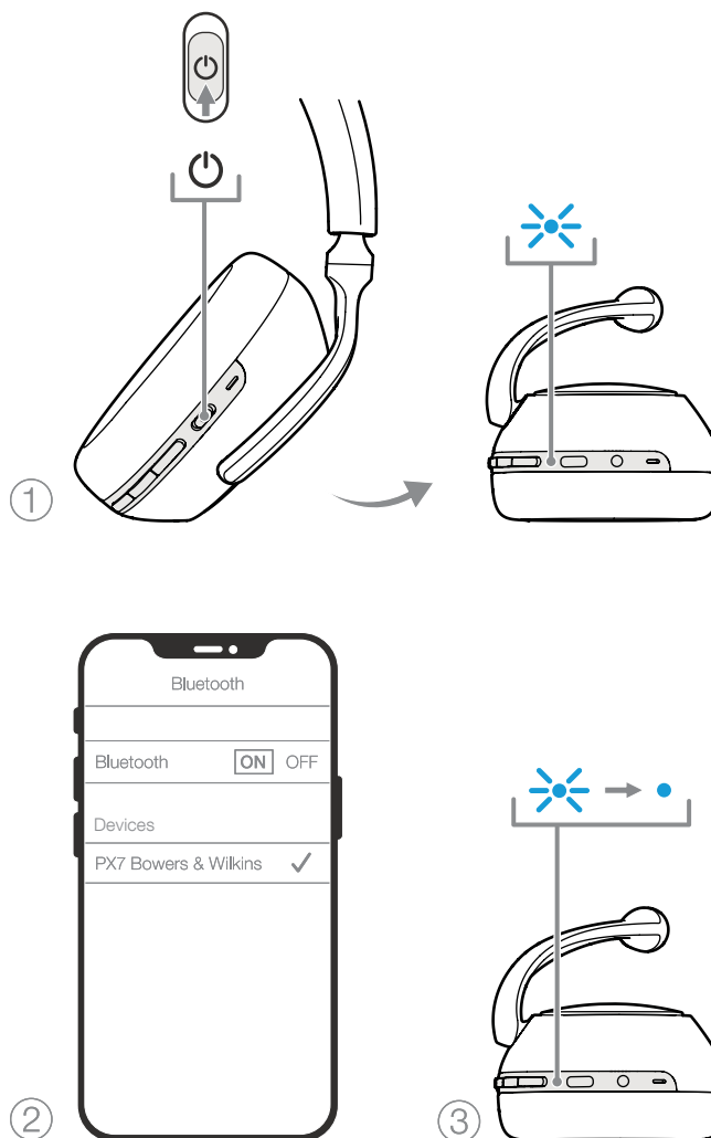
Figura 7 Abbinamento Bluetooth
